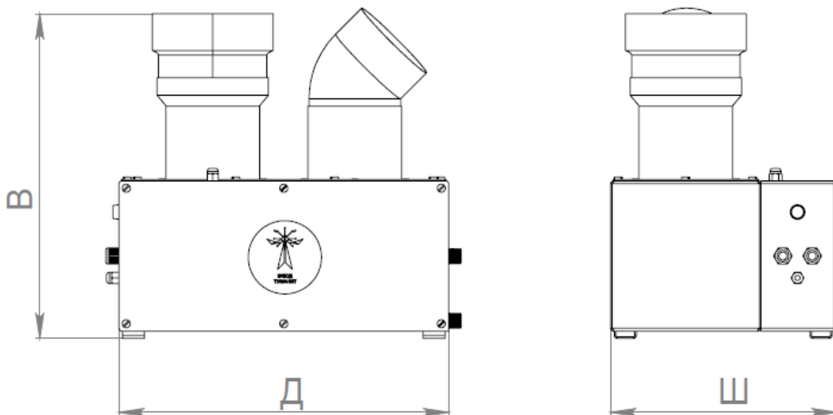
Рис.1 Модуль генерации
